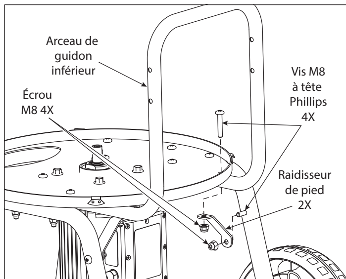
Figure 4 - Étape 9
