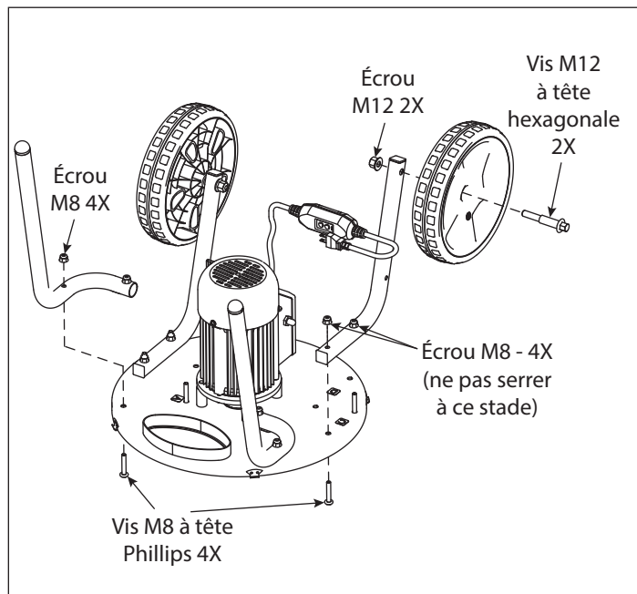
Figure 3 - Étapes 7 et 8
