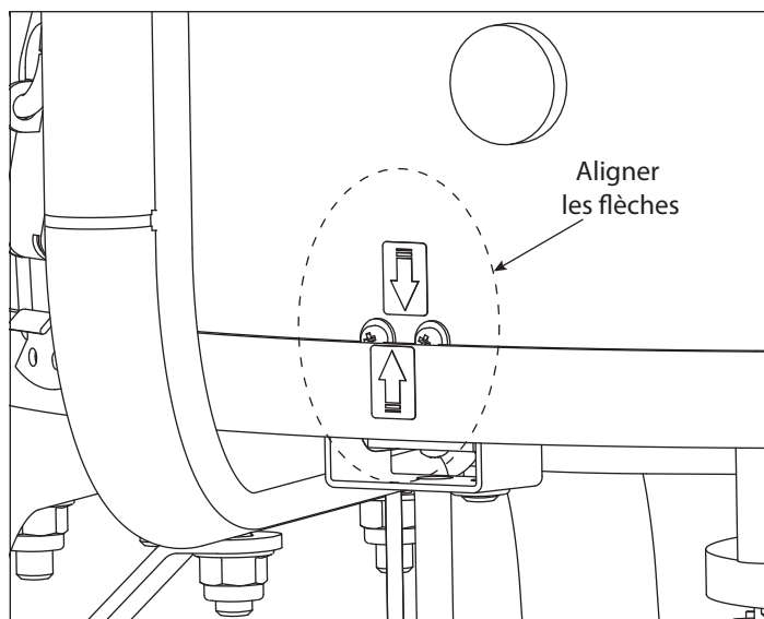
Figure 7 - Étape 14
